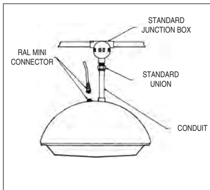
Rigid Pendant with Mini Receptacle
